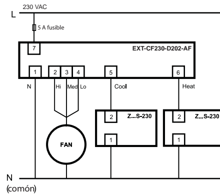
Control On/Off, con resorte de retorno de 2 cables
